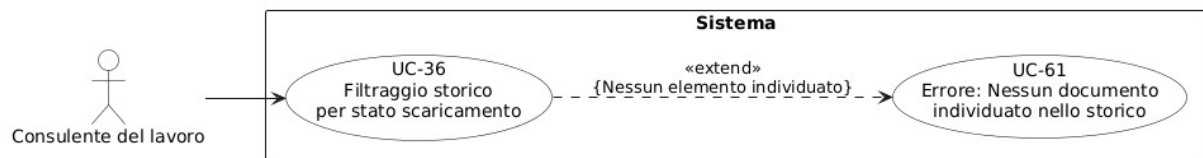
Figura 50: Diagramma del caso d'uso UC-36: Filtraggio storico per stato scaricamento
