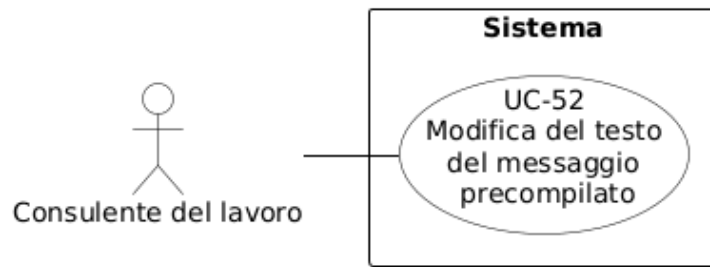
Figura 84: Diagramma del caso d'uso UC-52: Modifica del testo del messaggio precompilato
