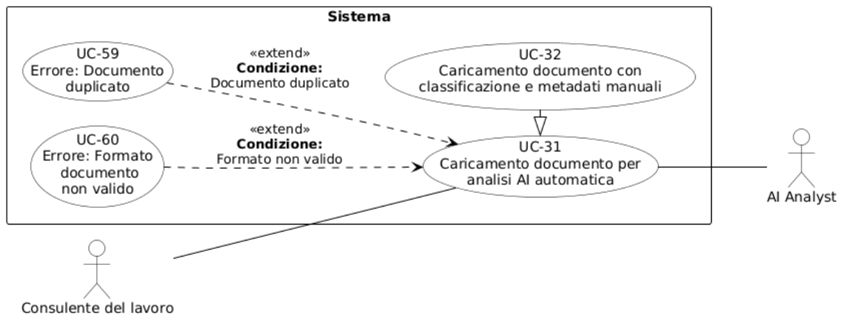
Figura 41: Diagramma del caso d'uso UC-31: Caricamento di un singolo documento per l'analisi AI automatica
