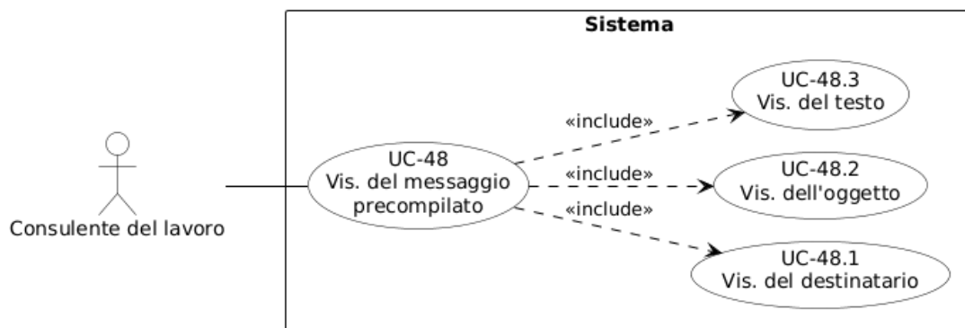
Figura 77: Diagramma del caso d'uso UC-48: Visualizzazione del messaggio precompilato
