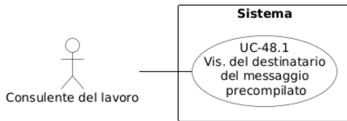
Figura 78: Diagramma del caso d'uso UC-48.1: Visualizzazione del destinatario
